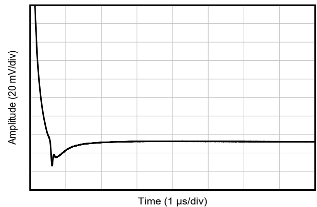
图 5-48. 稳定时间
