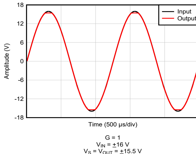
图 6-4. 无相位反转
