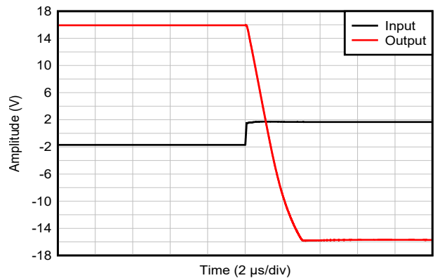
图 5-42. 正过载恢复
