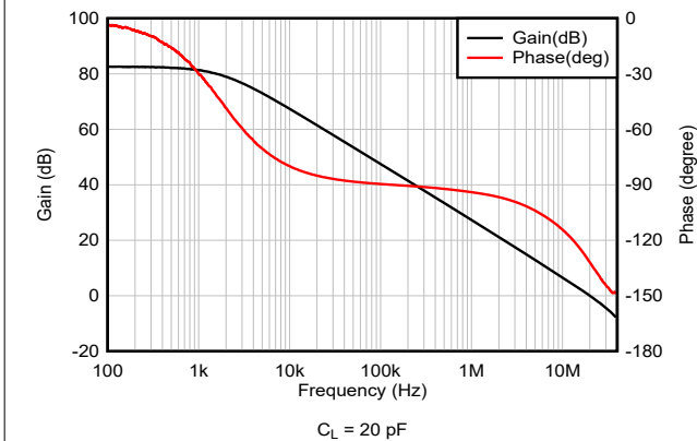
图 5-9. 开环增益和相位与频率间的关系
