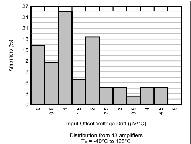
图 5-2. 失调电压漂移分配
