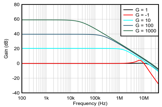
图 5-10. 闭环增益与频率间的关系
