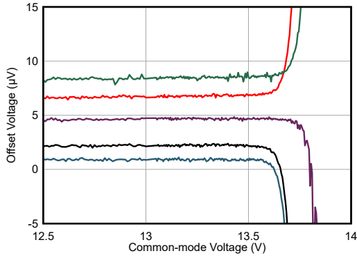
图 5-13. 在高电源电压下失调电压与 V_{CM} 间的关系
