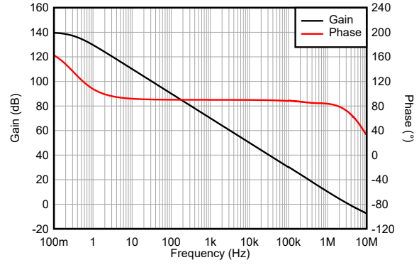
图 5-14. 开环增益和相位与频率间的关系
