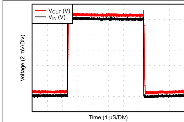
图 5-37. 负过载恢复
