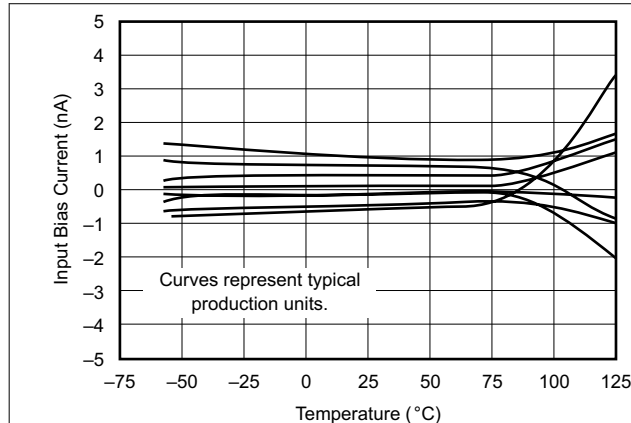
图 7-6. OPA2277 输入偏置电流
