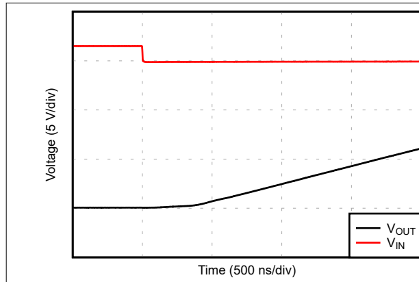
图 5-37. 负过载恢复
