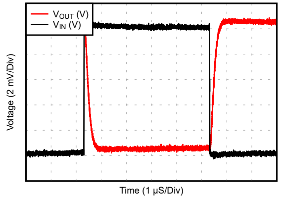
图 5-38. 建立时间
