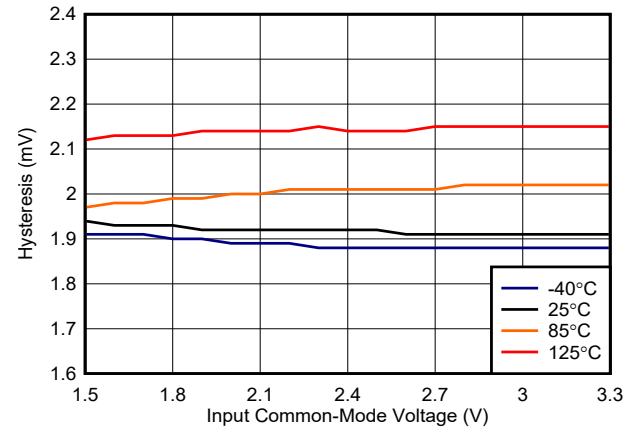
图 6-6. TLV3801 Hysteresis vs. Common-Mode, 3.3 V
