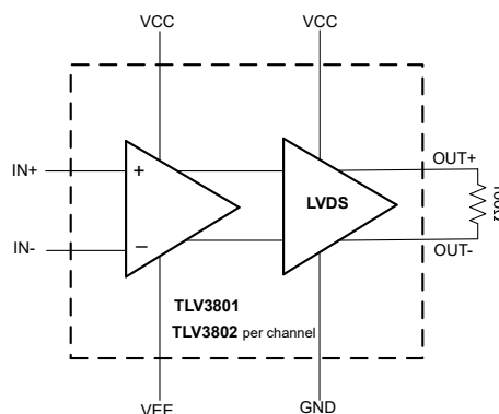
功能方框图
