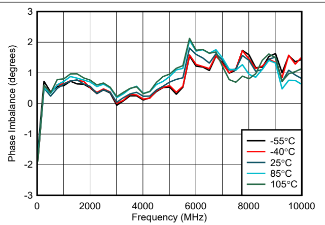
图 5-32. 相位不平衡
