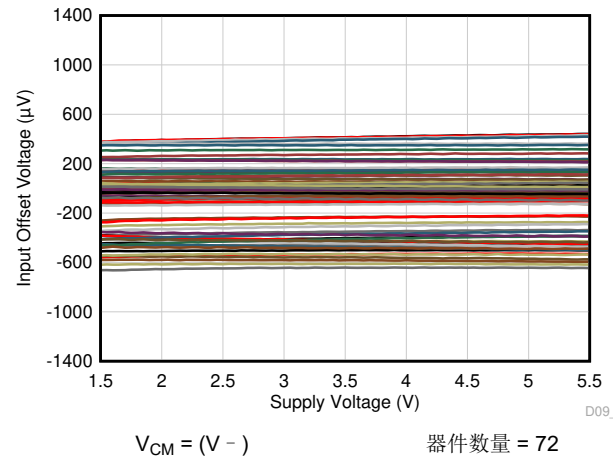
图 6-12. 偏移电压与电源电压间的关系
