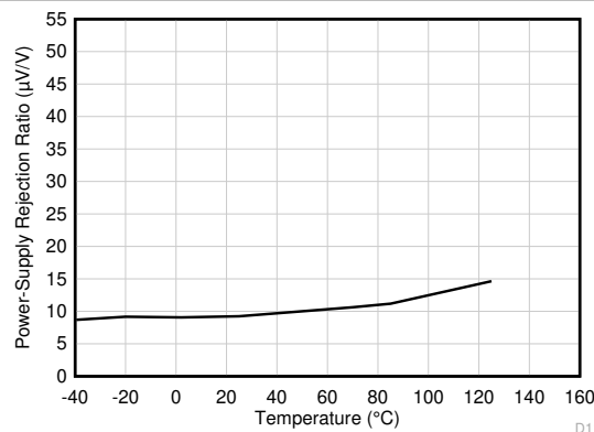
图 6-26. 直流 PSRR 与温度间的关系
