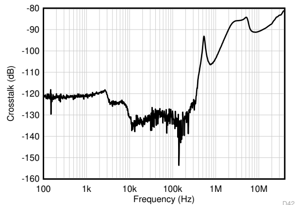
图 6-57. 通道隔离
