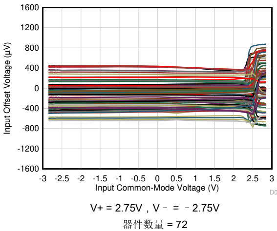
图 6-9. 失调电压与共模间的关系
