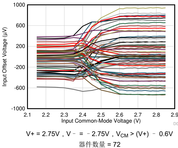
图 6-11. 失调电压与共模间的关系
