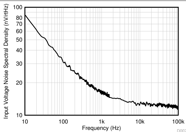
图 6-30. 输入电压噪声频谱密度
