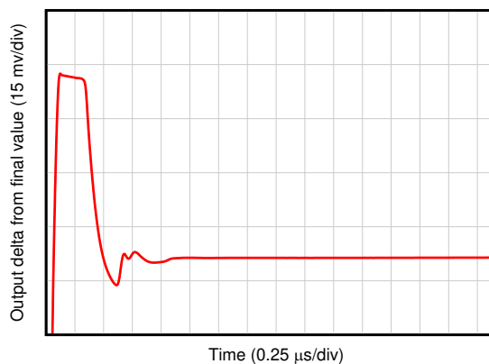
图 6-46. 大信号阶跃响应
