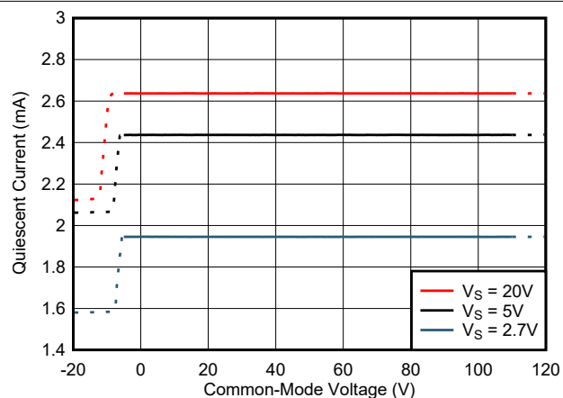
图 7-32. 静态电流与共模电压间的关系
