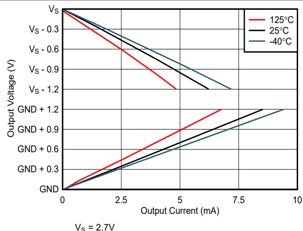
图 7-22. 输出电压与输出电流间的关系
