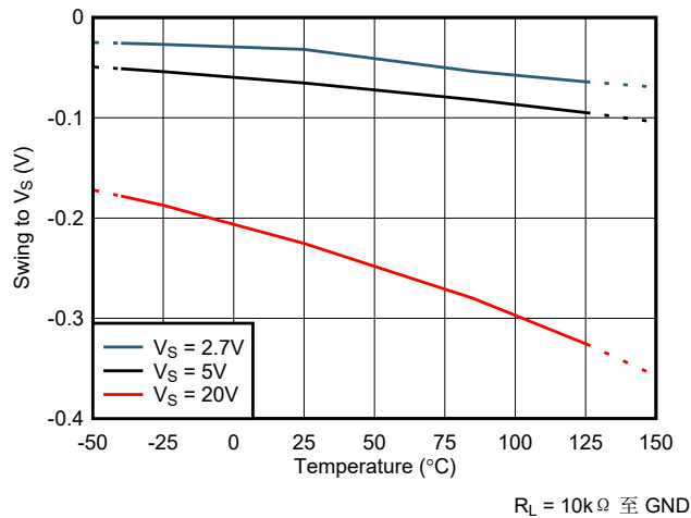
图 7-25. 电源摆幅与温度间的关系
