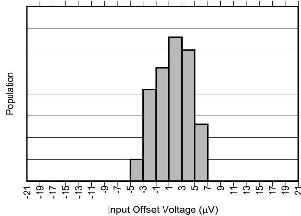
图 7-1. INA296A1 输入失调电压产生分布图
