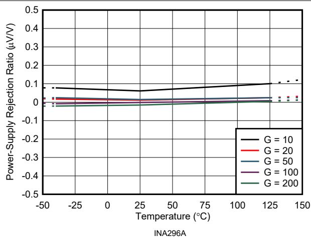
图 7-14. 电源抑制比与温度间的关系
