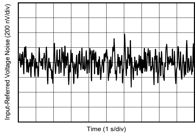
图 7-28. 0.1Hz 至 10Hz 电压噪声
