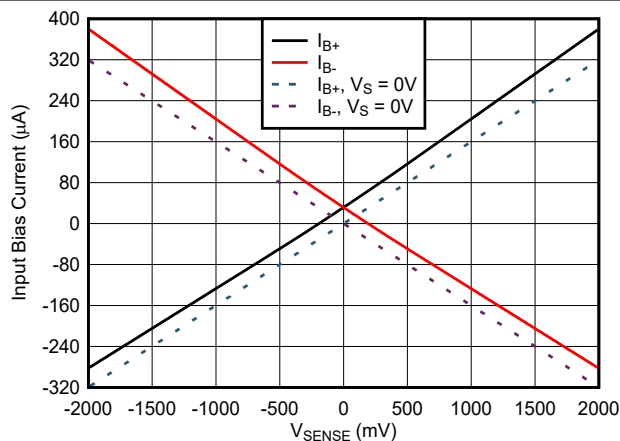
图 7-18. INA296x1 输入偏置电流与 V_{\text{SENSE}} 间的关系
