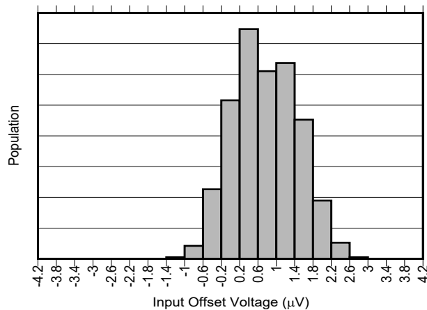
图 7-3. INA296A3 和 INA296A4 输入失调电压产生分布图
