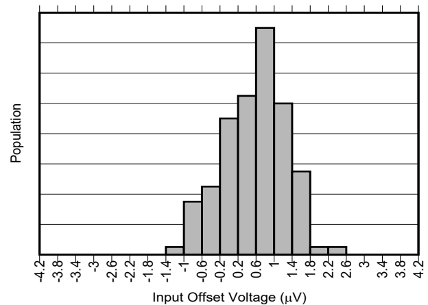
图 7-4. INA296A5 输入失调电压产生分布图
