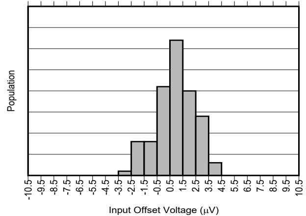
图 7-2. INA296A2 输入失调电压产生分布图
