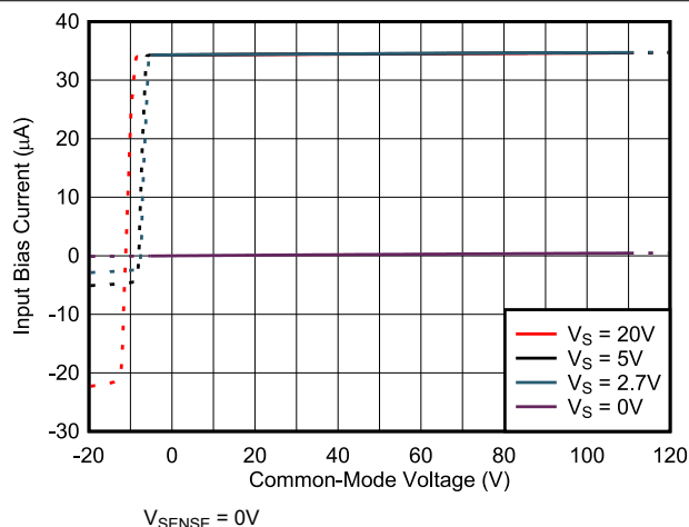
图 7-16. 输入偏置电流与共模电压间的关系
