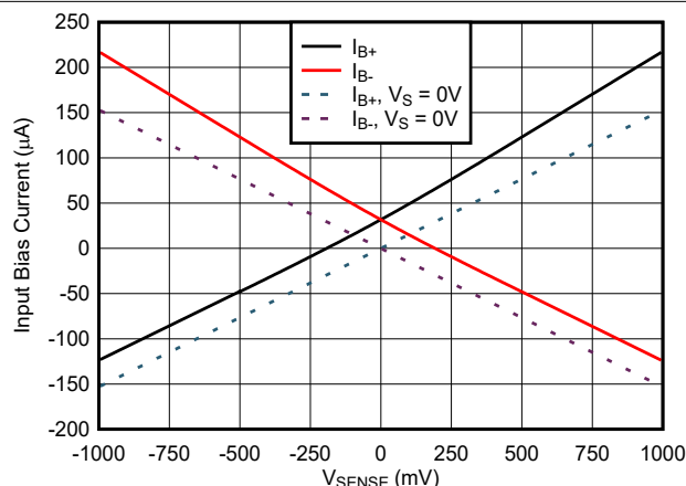
图 7-19. INA296x2 输入偏置电流与 V_{\text{SENSE}} 间的关系
