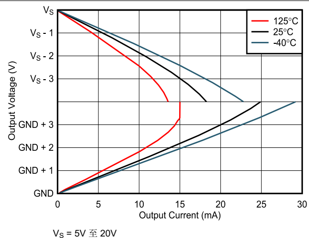
图 7-23. 输出电压与输出电流间的关系
