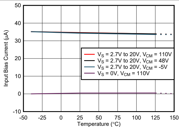
图 7-17. 输入偏置电流与温度间的关系
