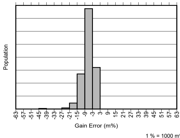
图 7-12. 所有增益 INA296B 增益误差产生分布图
