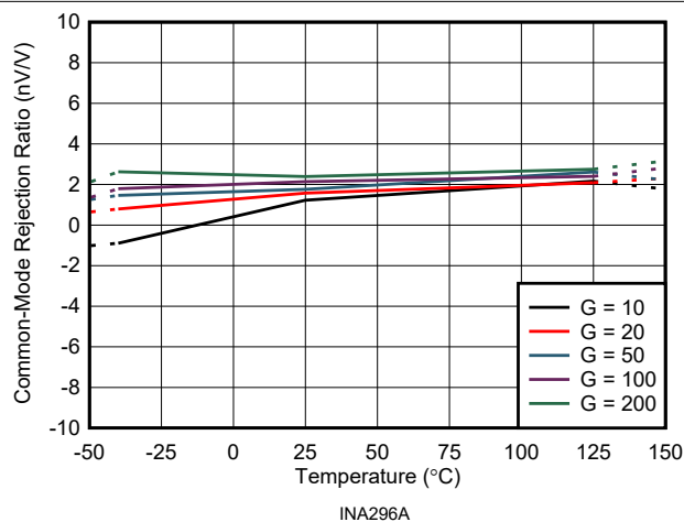
图 7-7. 共模抑制比与温度间的关系
