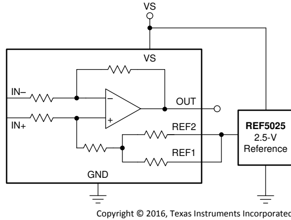
图 8-4. 外部基准输出
