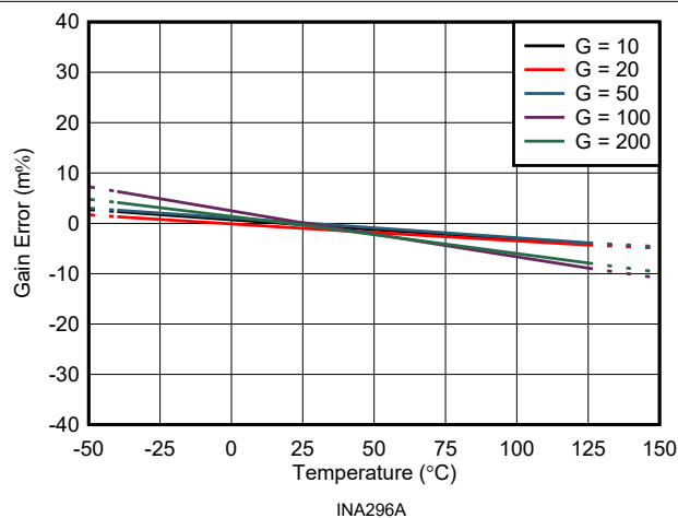
图 7-13. 增益误差与温度间的关系
