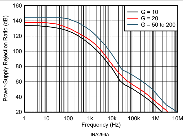
图 7-15. 电源抑制比与频率间的关系
