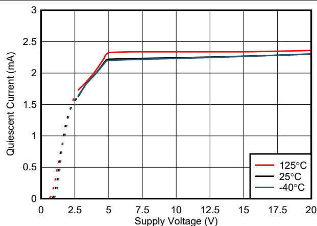
图 7-31. 静态电流与电源电压间的关系
