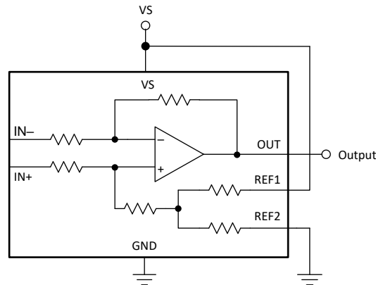
图 8-5. 1/2 V_s 电压输出
