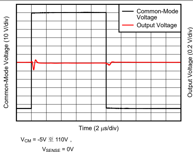
图 7-33. 共模电压快速瞬态脉冲
