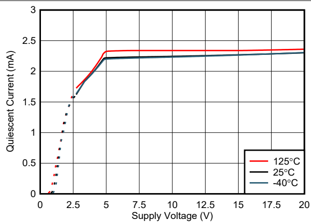
图 6-31. 静态电流与电源电压间的关系
