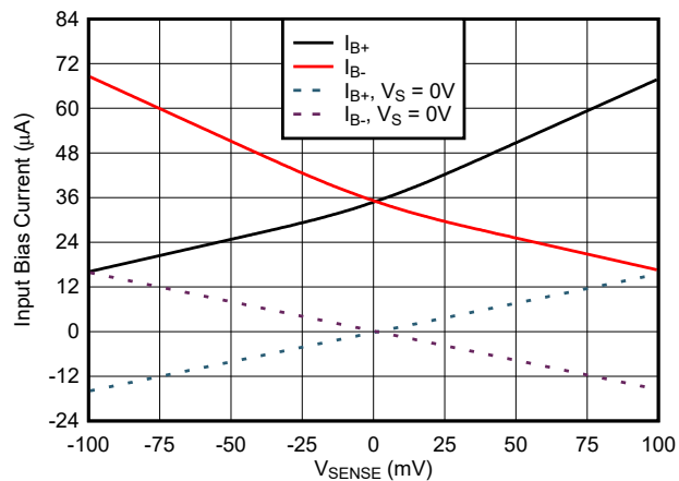
图 6-21. INA296x5-Q1 输入偏置电流与 V_{\text{SENSE}} 间的关系
