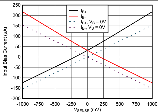
图 6-19. INA296x2-Q1 输入偏置电流与 V_{\text{SENSE}} 间的关系
