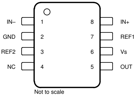
图 5-1. INA296x-Q1 : DDF 封装 8 引脚 SOT-23 顶视图
