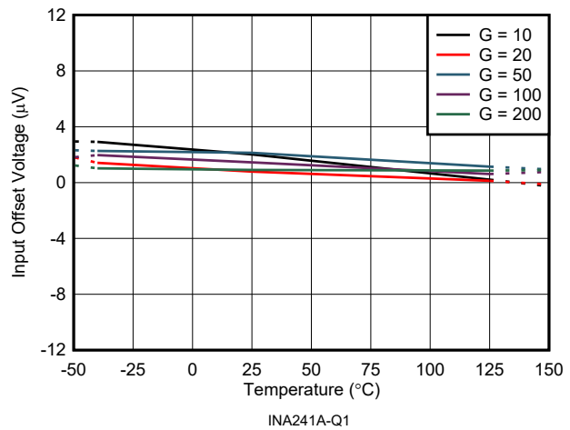
图 6-6. 输入失调电压与温度间的关系
