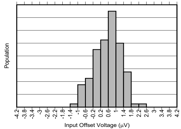
图 6-4. INA241A5-Q1 输入失调电压产生分布图
