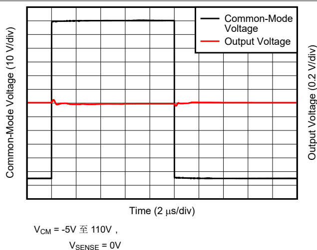
图 6-33. 共模电压快速瞬态脉冲
