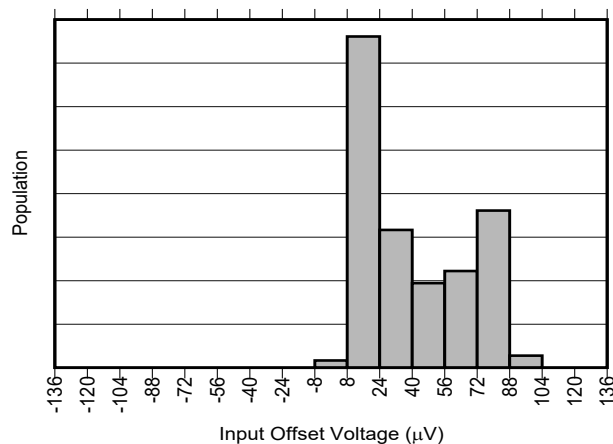
图 6-3. INA241A3-Q1 和 INA241A4-Q1 输入失调电压产生分布图
