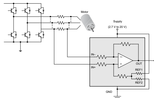
典型应用 - 直列式电机控制
