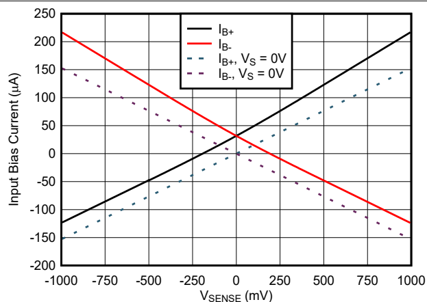
图 6-19. INA241x2-Q1 输入偏置电流与 V_{\text{SENSE}} 间的关系
