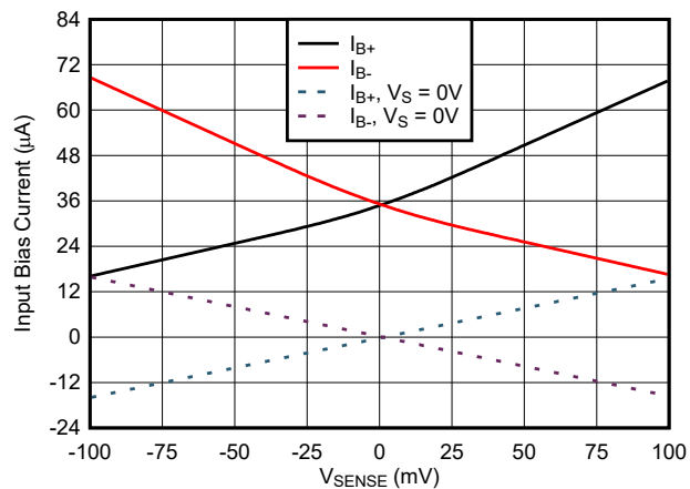
图 6-21. INA241x5-Q1 输入偏置电流与 V_{\text{SENSE}} 间的关系
