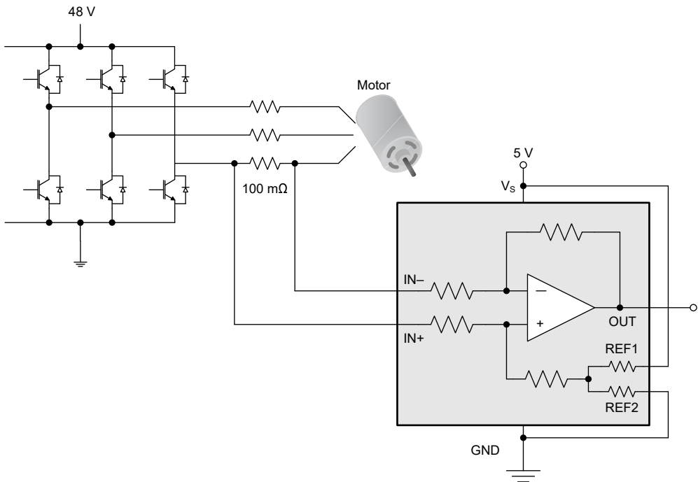
图 8-1. 直列式电机应用电路
