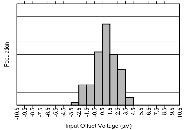
图 6-2. INA241A2-Q1 输入失调电压产生分布图
