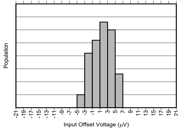
图 6-1. INA241A1-Q1 输入失调电压产生分布图
