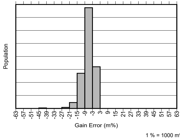
图 6-12. 所有增益 INA241B-Q1 增益误差产生分布图
