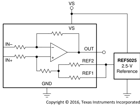
图 7-5. 外部基准输出
